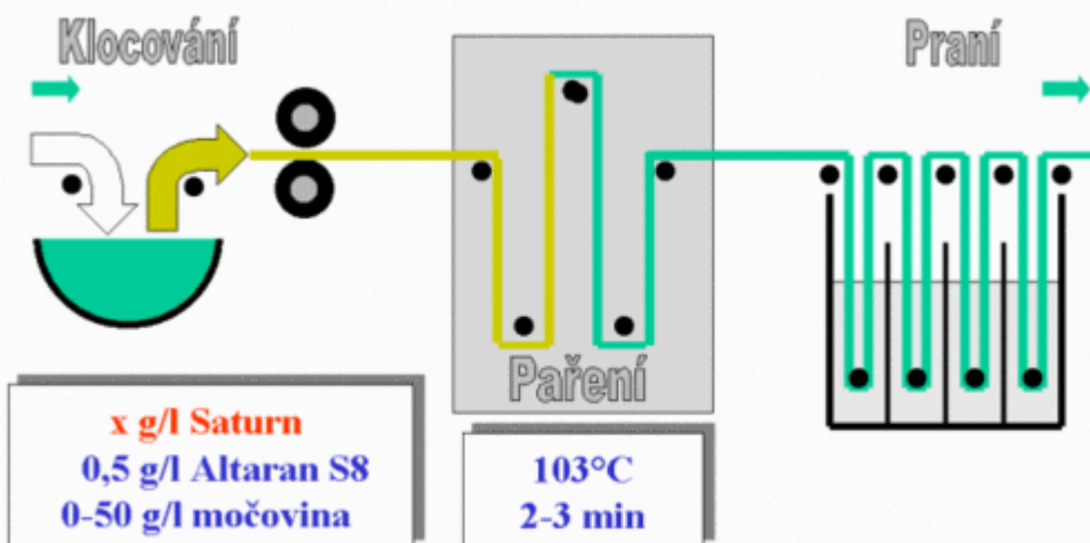
Klocovací postup Pad - Batch ●
