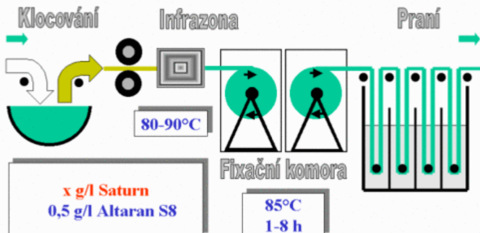
Klocovací postup Pad - Steam ●
